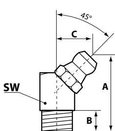
15 940 M 6 x 1-VA-SK-SW 9 A: 23,5 B: 5,5 C: 10,5
