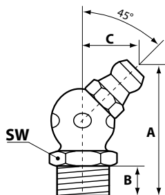
15 107 140 M 6 x 1-VZ-SK-SW 9 A: 23,5 B: 5,5 C: 10,5
